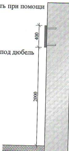
Рис.3. Узел крепления информационной пластины к фасаду
