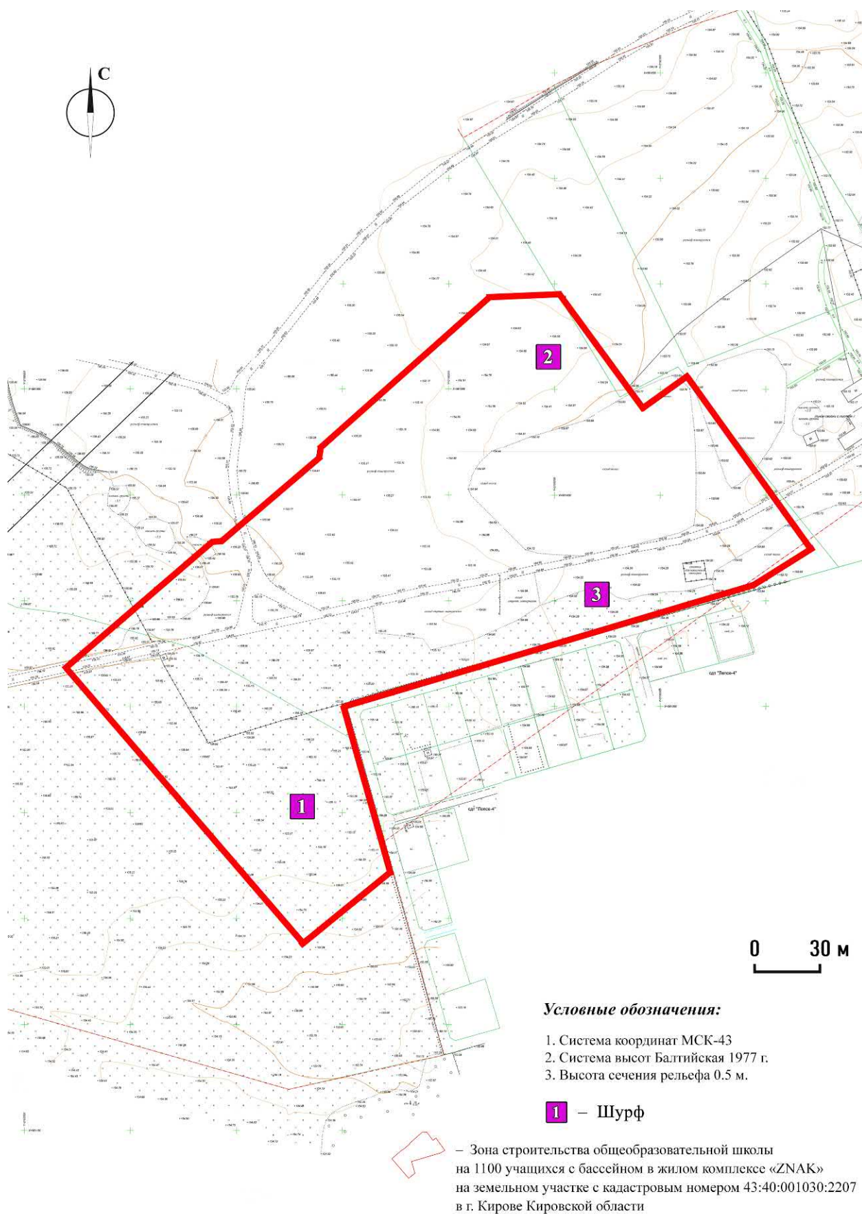
Рис. 15. Инженерно-топографический план с обозначением исследуемой территории и заложенных шурфа в зоне строительства общеобразовательной школы на 1100 учащихся с бассейном в жилом комплексе «ZNAK» на земельном участке с кадастровым номером 43:40:001030:2207 в г. Кирове Кировской области.
