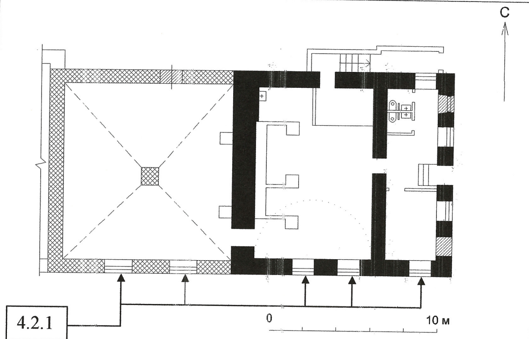
план подвального этажа
