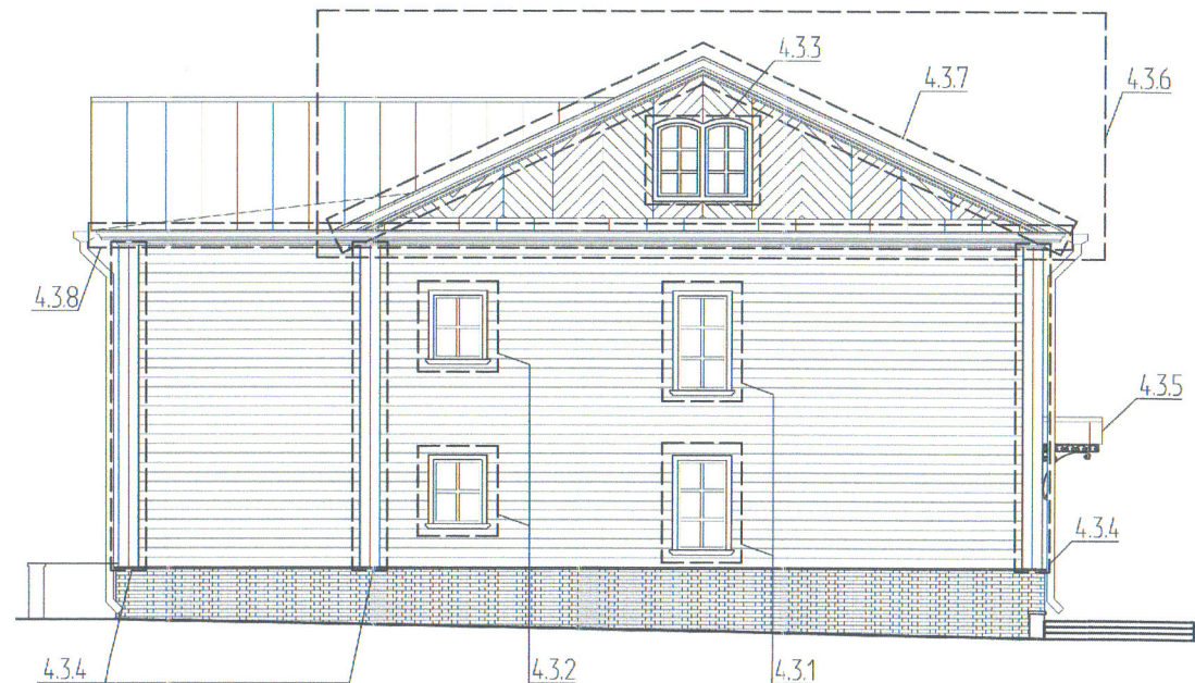
Восточный фасад
