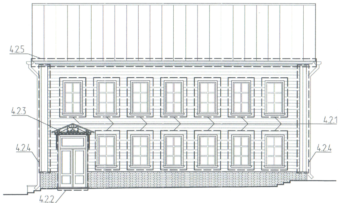
Северный фасад
