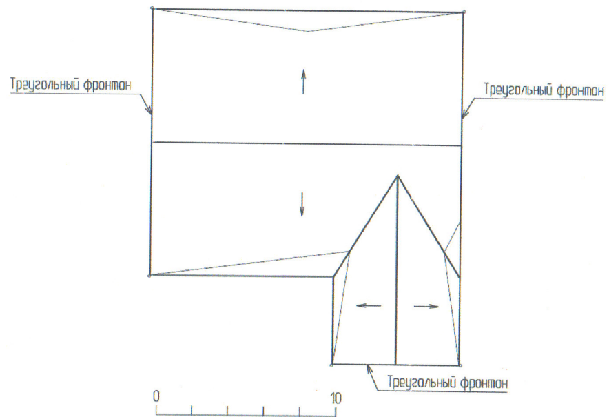
План кровли
