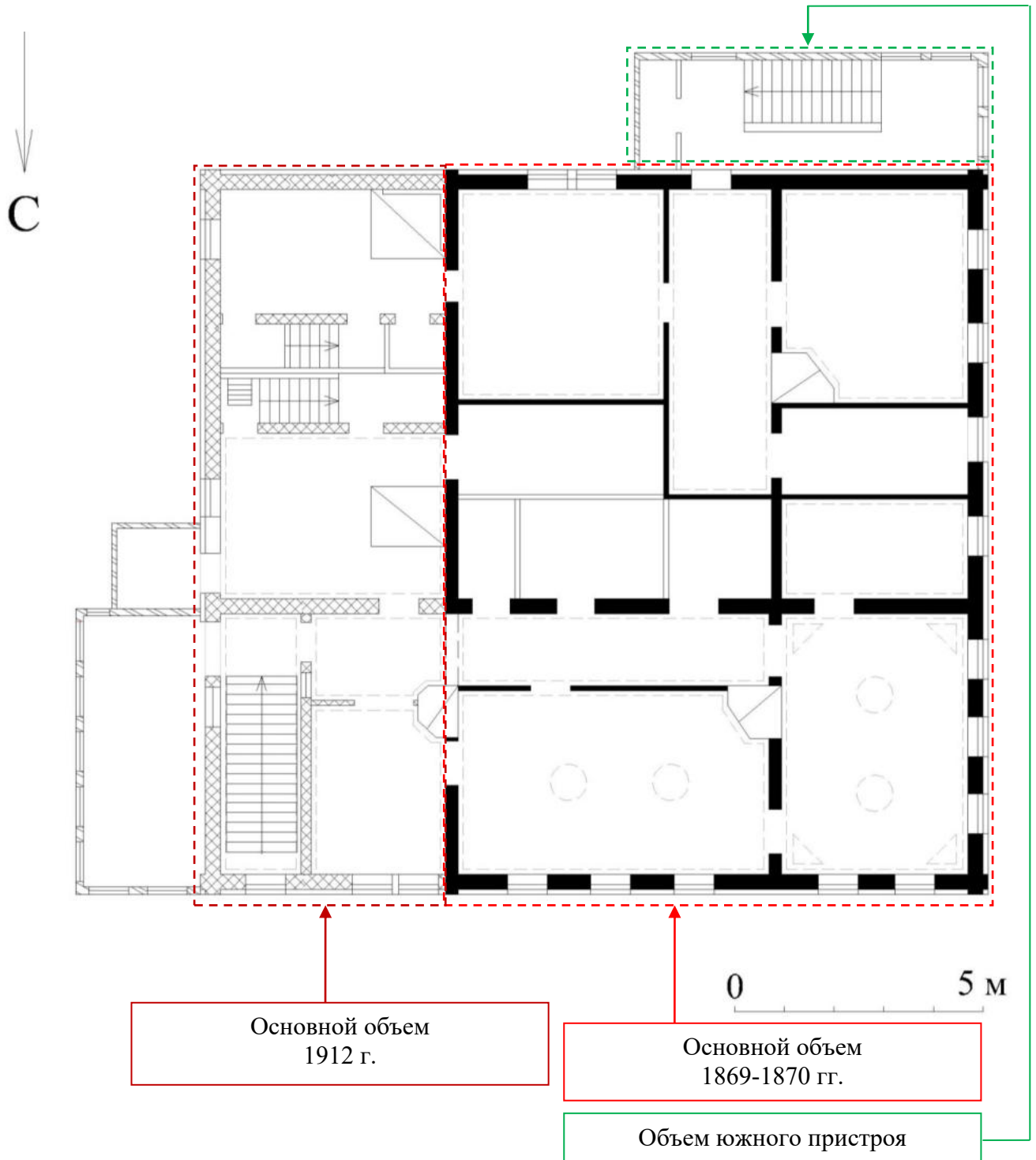
Илл. 36. Схема объемов, включенных в Предмет охраны на плане второго этажа.
