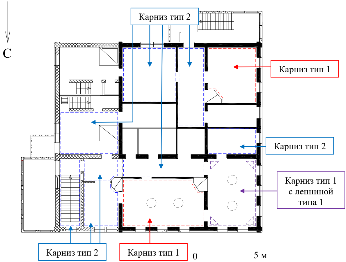
Илл. 31. Схема расположения карнизов и потолочных розеток на плане второго этажа.
