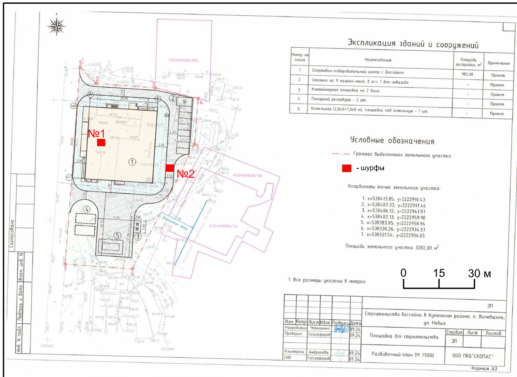
Рис. 6. Топографический план-схема с указанием участка проведения работ на земельных участках, выделенных под строительство объекта «Строительство бассейна в пос. Вичевщина, Куменский район, Кировская область» на з/у с кадастровым номером 43:14:040101:2534, расположенном по адресу: Кировская область, Куменский район, п. Вичевщина, ул. Новая, з/у 6 и заложенных шурфов в 2025 г.
