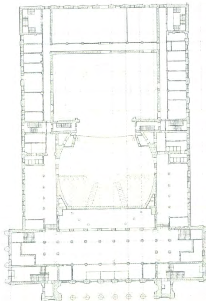
План схема 1-ого этажа
