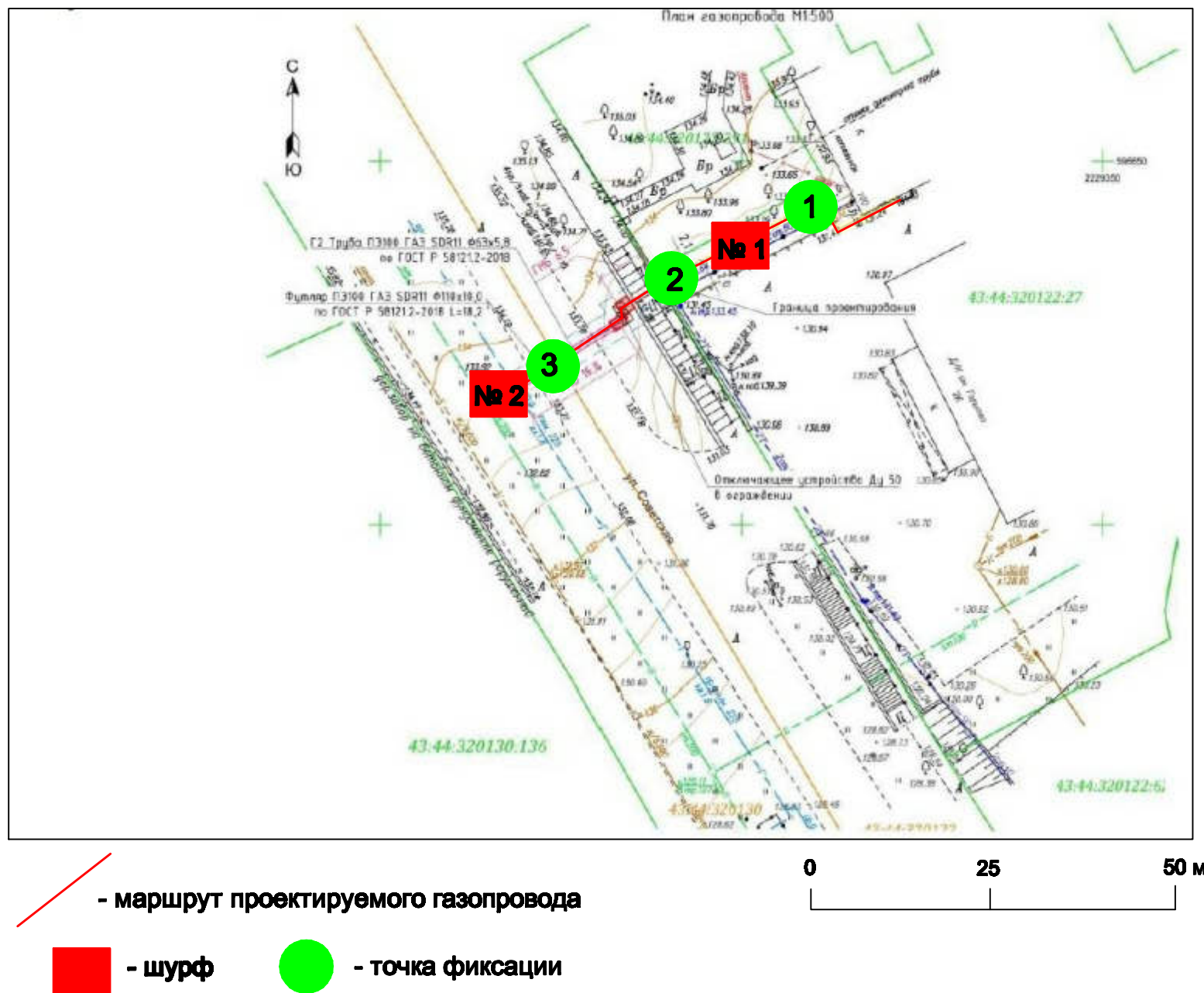
Рис. 5. Топографический план маршрута проектируемого газопровода к дому культуры и мест закладки шурфов в г. Слободском Слободского района Кировской области в 2025 г.
