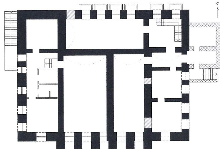
план цокольного этажа
