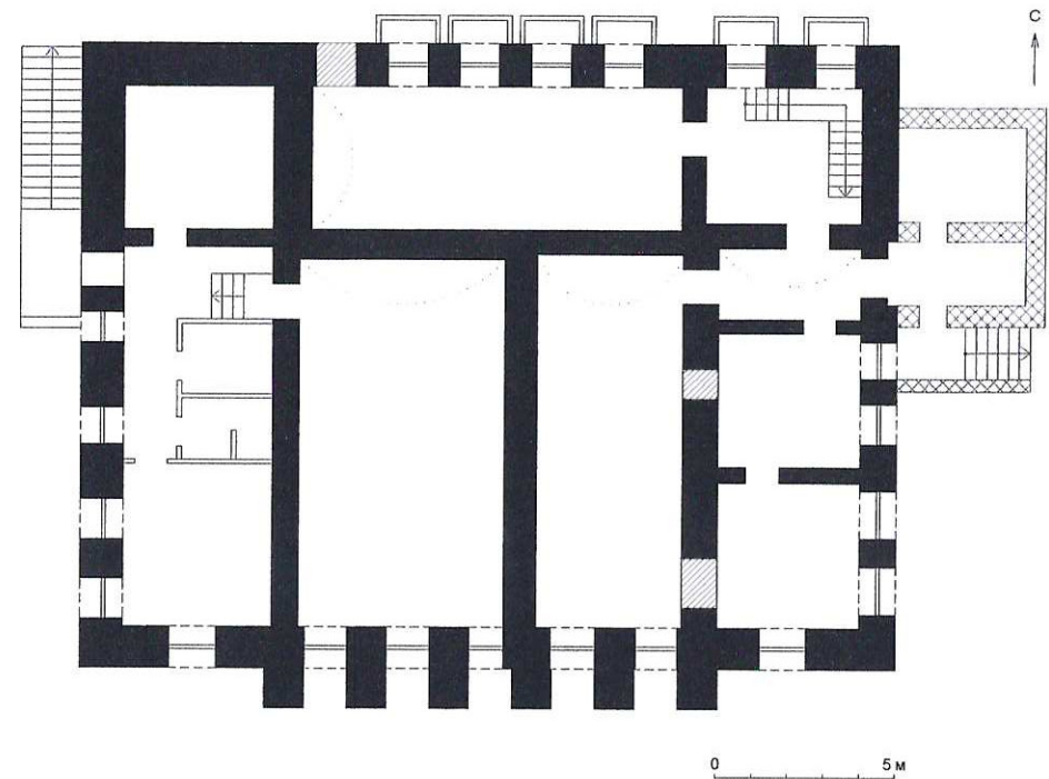
план цокольного этажа
